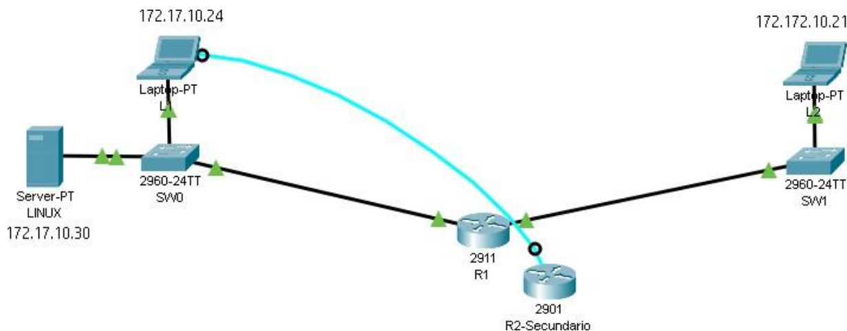
Figura1. Posible RED LAN Conexión de 2 Centros Universitarios
